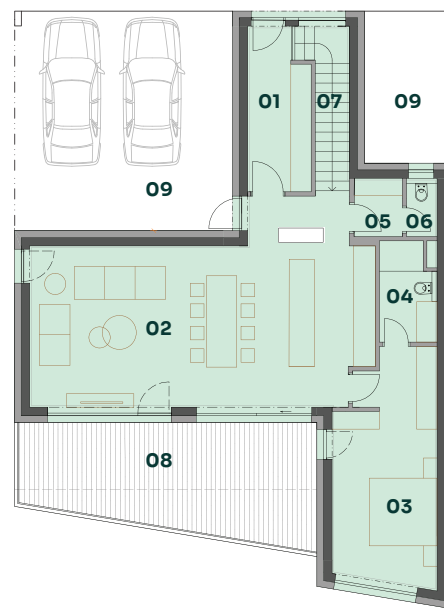
Půdorys 1.NP
