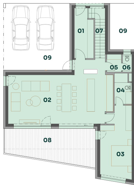
Půdorys 1.NP
